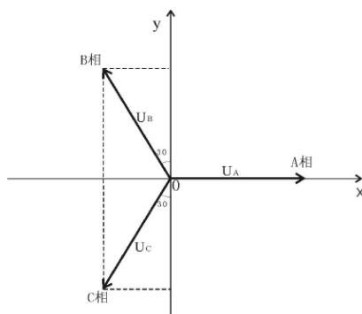
图 a 对地电压计算图
