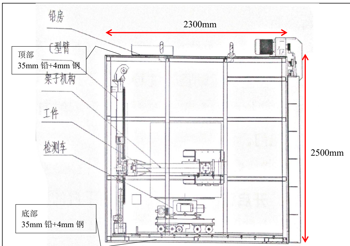
图 10-2 本项目装置主体左视图（视线自南向北）
