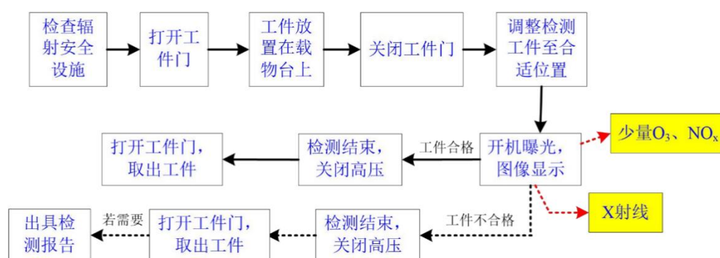
图 9-3 本项目 X 射线实时成像检测装置工作流程及产污环节分析示意图
