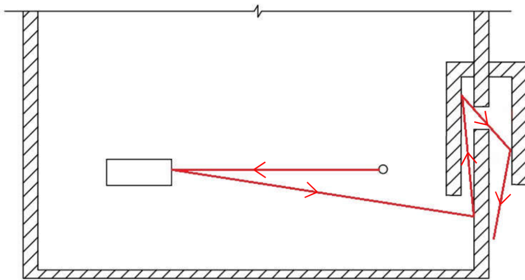
图 11-4 电缆孔散射示意剖面图
