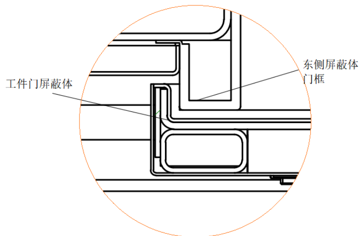
图 11-5 工件门门扣边示意图
