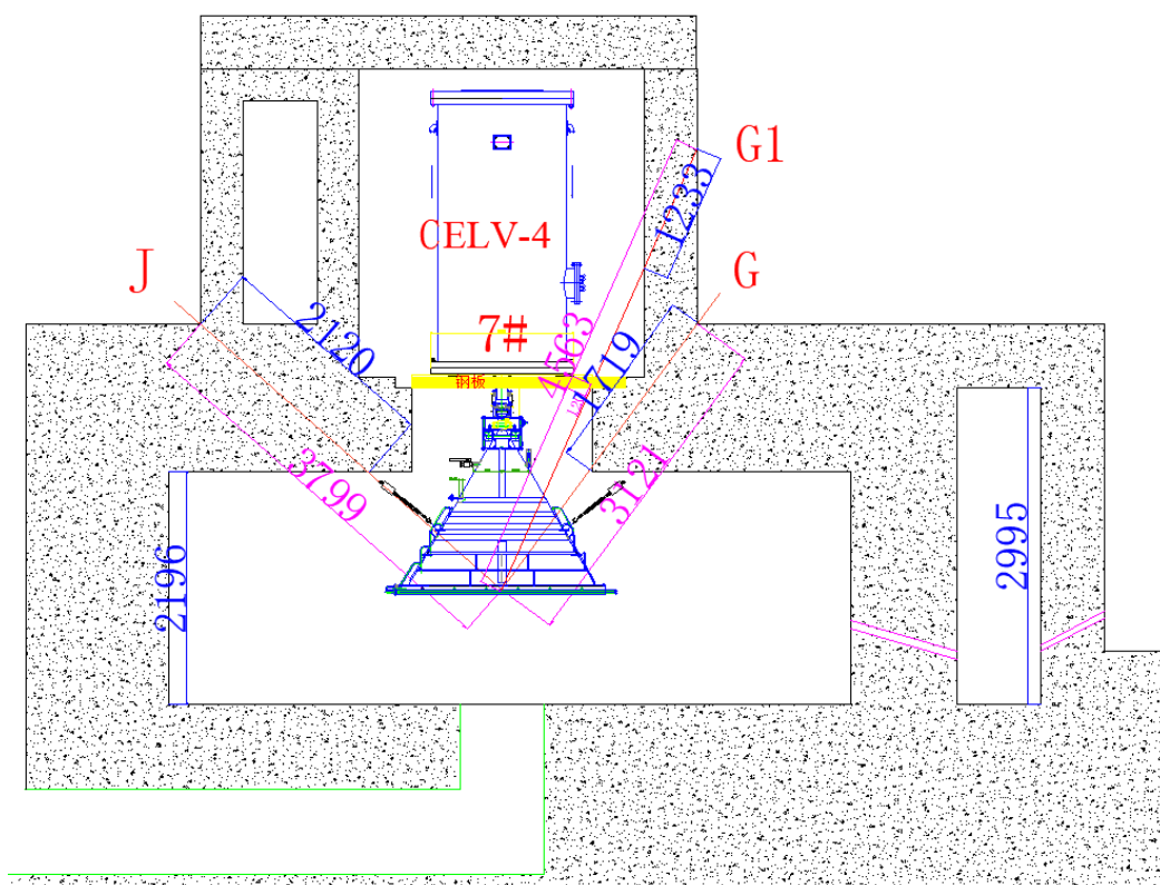
图 11-4 本项目加速器机房辐照室 X 射线直射到主机室周围屏蔽计算参考点位示意图 (南北向剖面)
