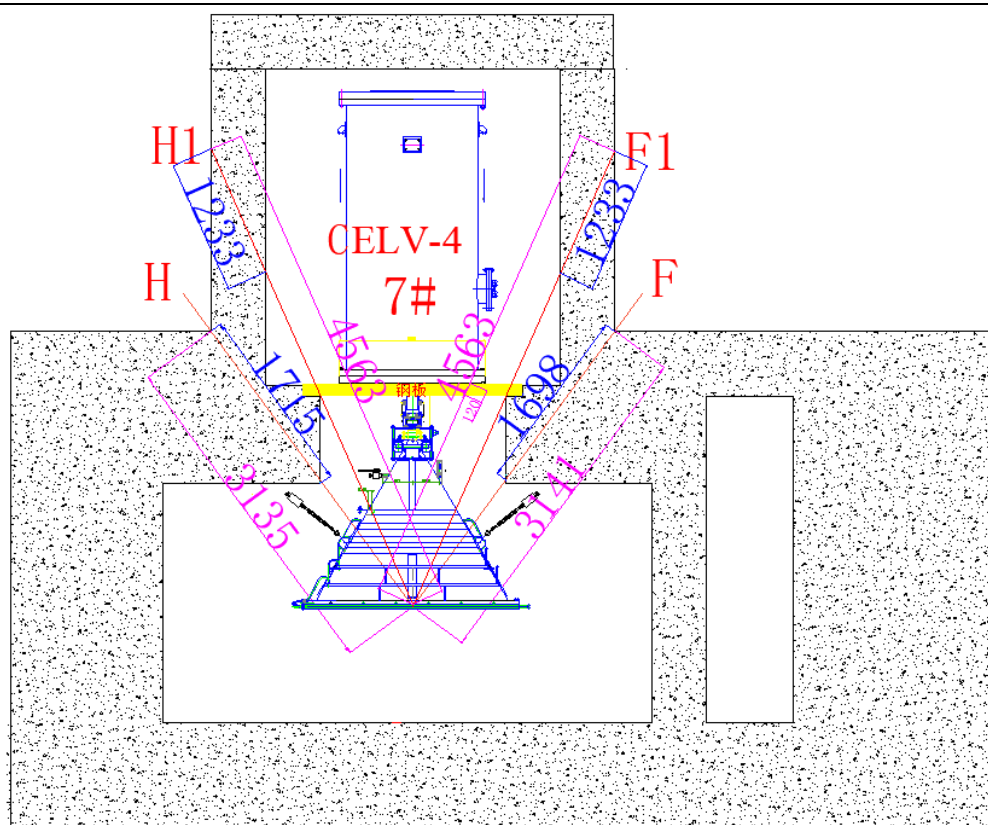
图 11-3 本项目加速器机房辐照室 X 射线直射到主机室周围屏蔽计算参考点位示意图 (东西向剖面)
