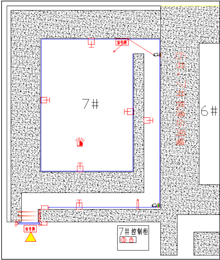
图 10-3 本项目加速器机房一层辐照室辐射安全装置布设示意图
