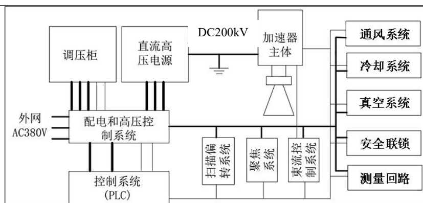
图 9-3 本项目 2 台电子加速器系统结构图
