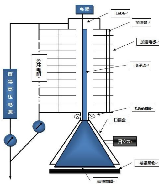
图 9-4 本项目 2 台电子加速器自屏蔽电子加速器辐照装置工作原理示意图
