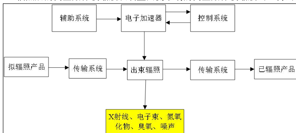
图 9-5 本项目 2 台加速器装置辐照加工工艺流程和主要产污环节图
