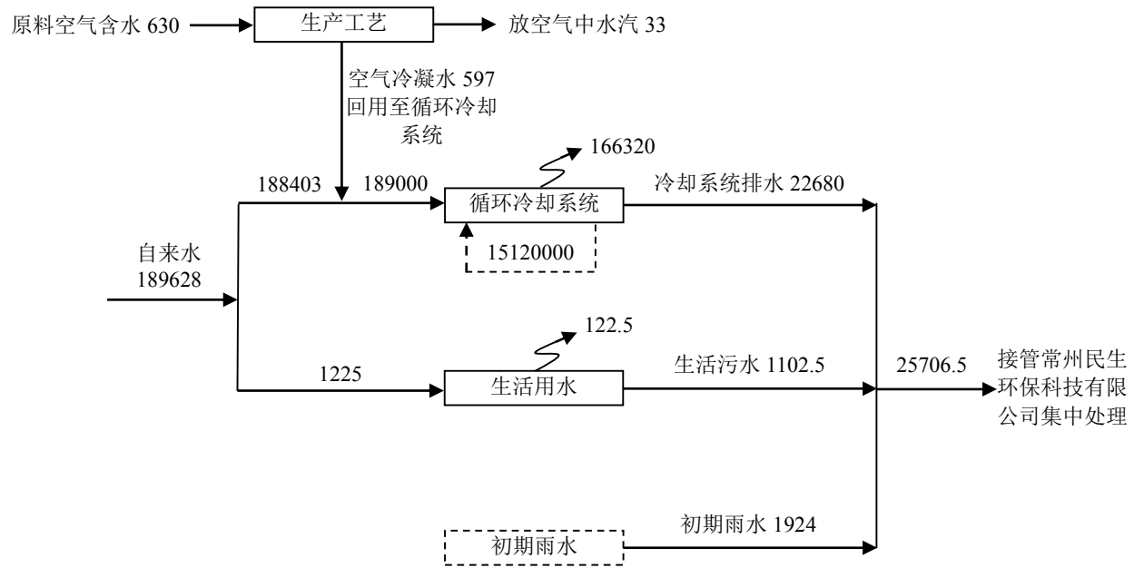
图 2-1 本项目水平衡图（单位：m³/a）
