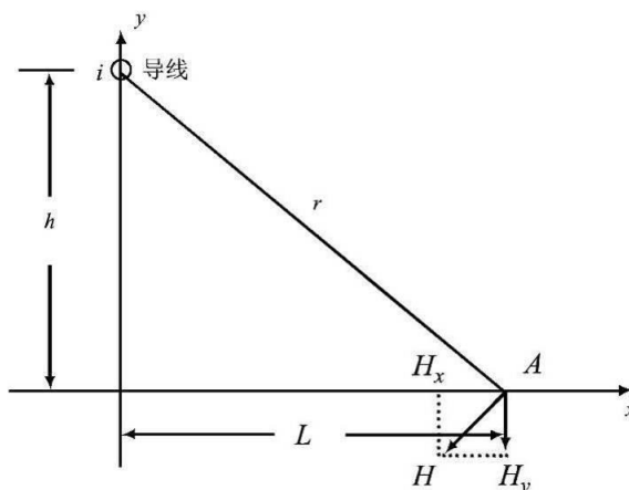
图 3.3-4 磁场向量图
