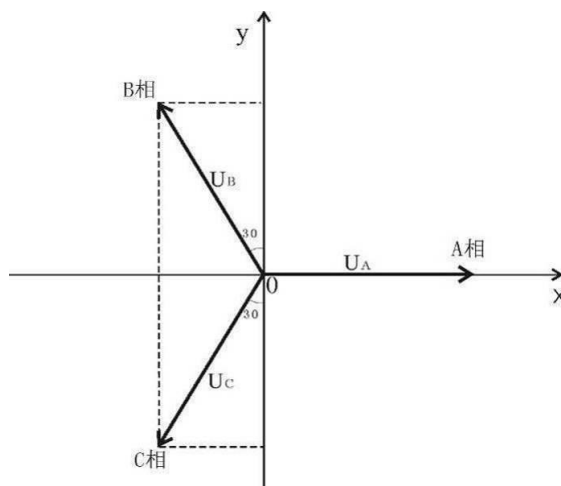
图 3.3-1 对地电压计算图
