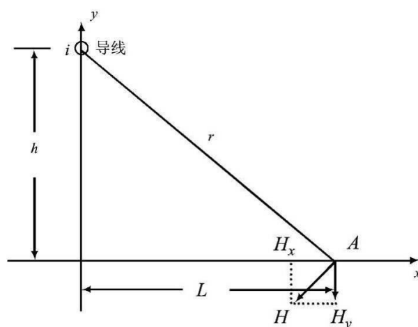
图 3.1-5 磁场向量图
