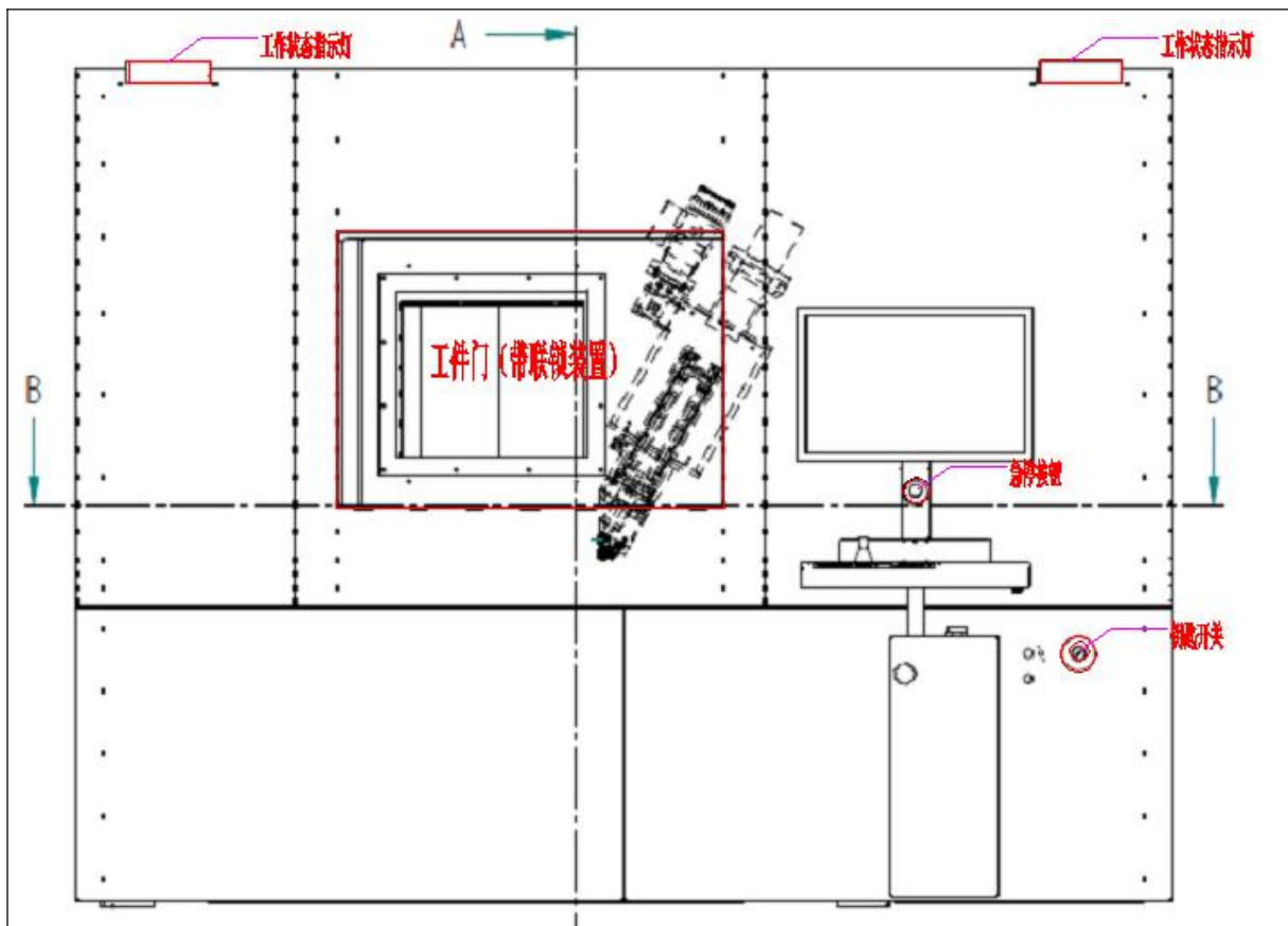
图 10-3 辐射安全措施分布图
