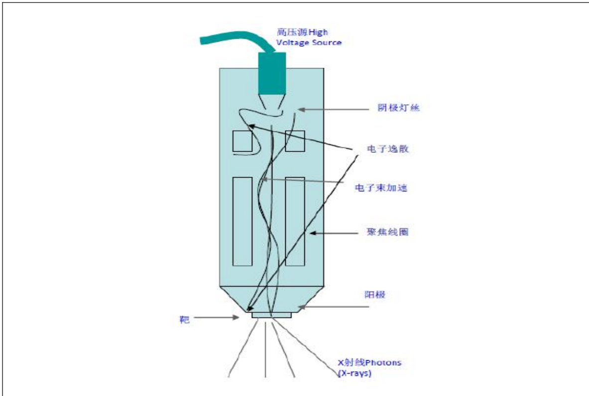
图 9-2 X 射线管结构图
