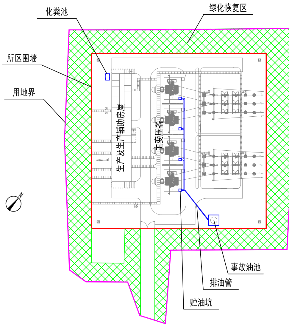
生态环境保护措施布置图
