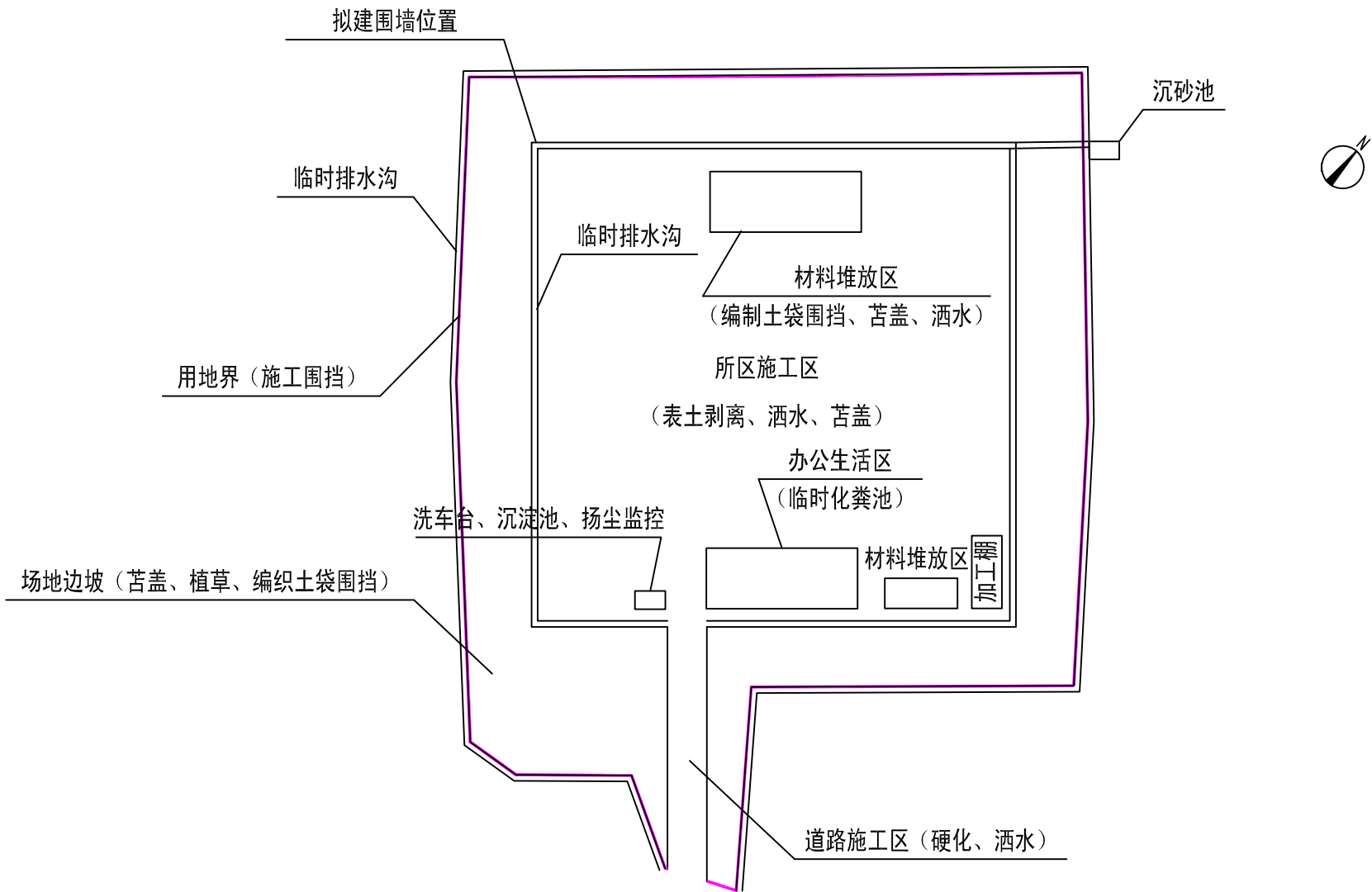
施工布置及环保措施布置图
