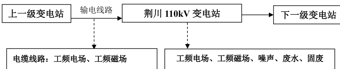
图 1 江苏常州荆川 110kV 输变电工程工艺流程及产污环节示意图
