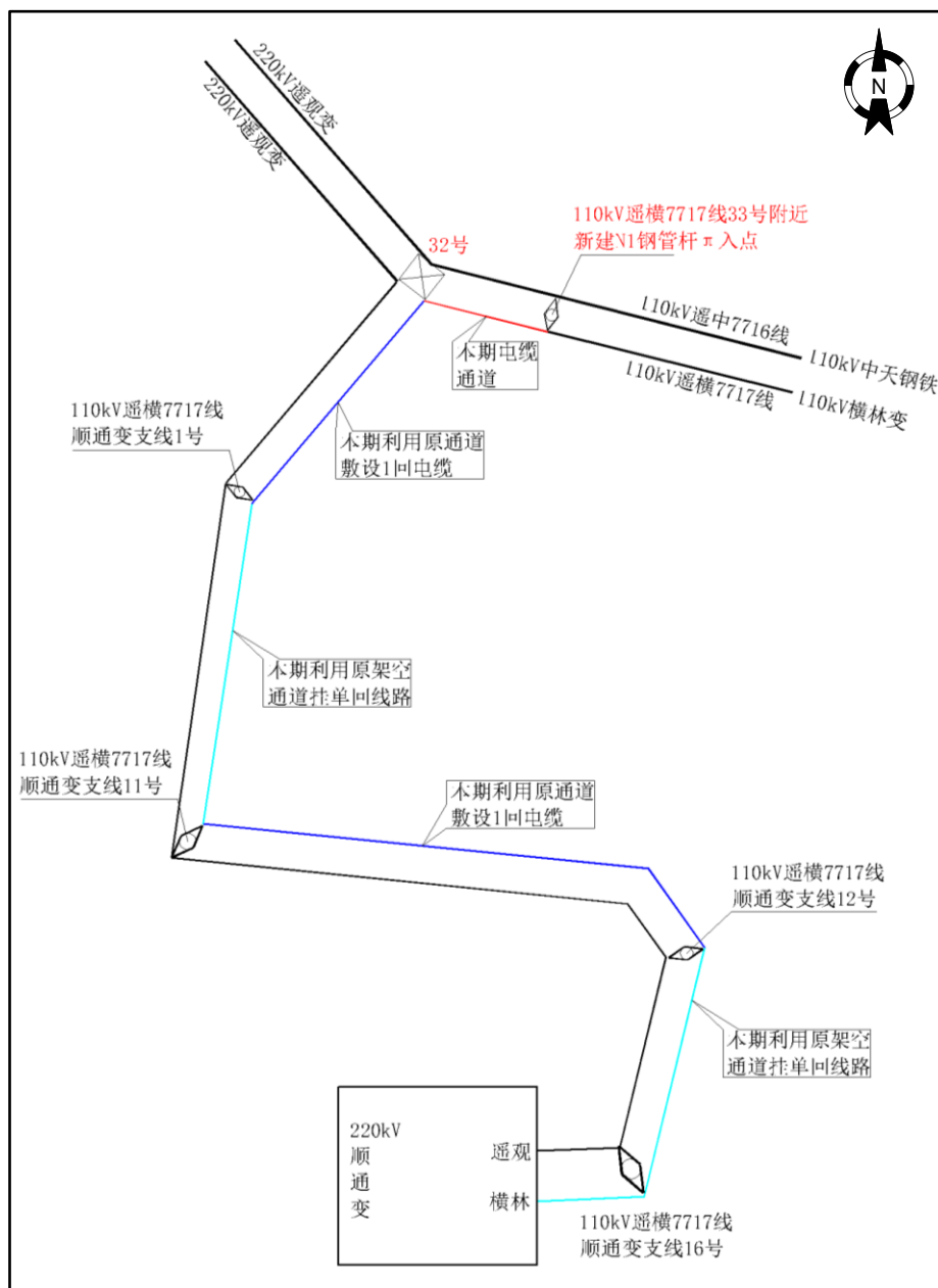
图 1 本工程接线示意图
