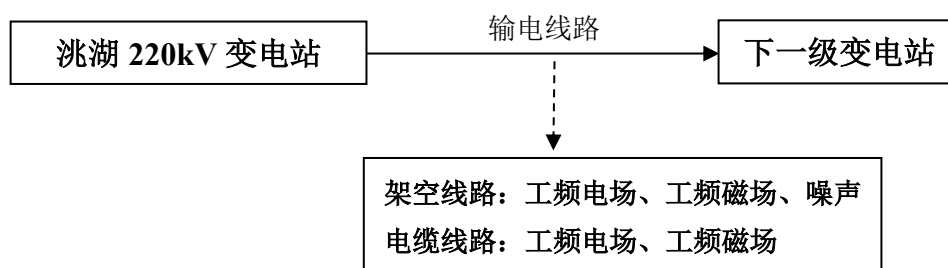
图 1 常州洮湖变至方麓变 110kV 线路工程工艺流程及产污环节示意图
