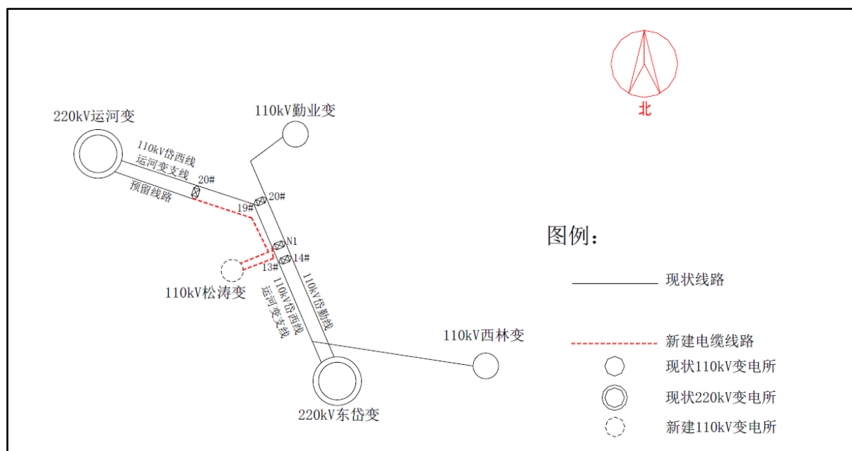
图 1 本工程线路接线示意图示意图
