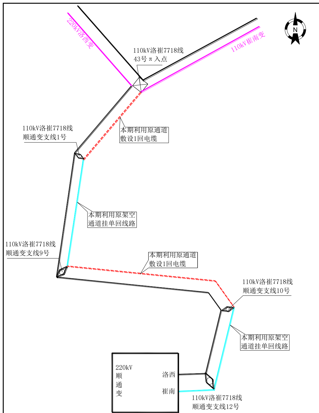
图 1 本工程接线示意图
